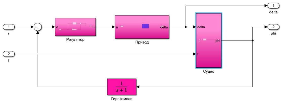
Рисунок 1 – Общая схема линейном система управления судна
