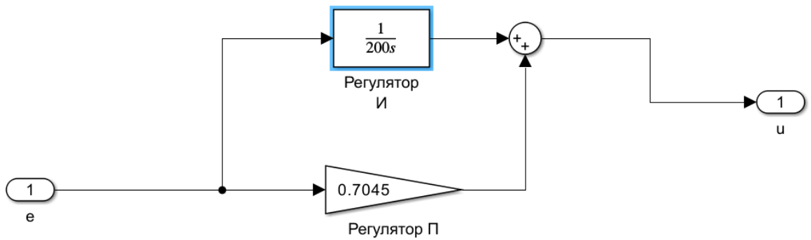
Рисунок 2 – Регулятор линейной схемы системы управления судна
